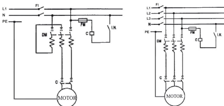
Obrázek 9 – schéma elektrozapojení protiproudu FLOW JET 3000™
