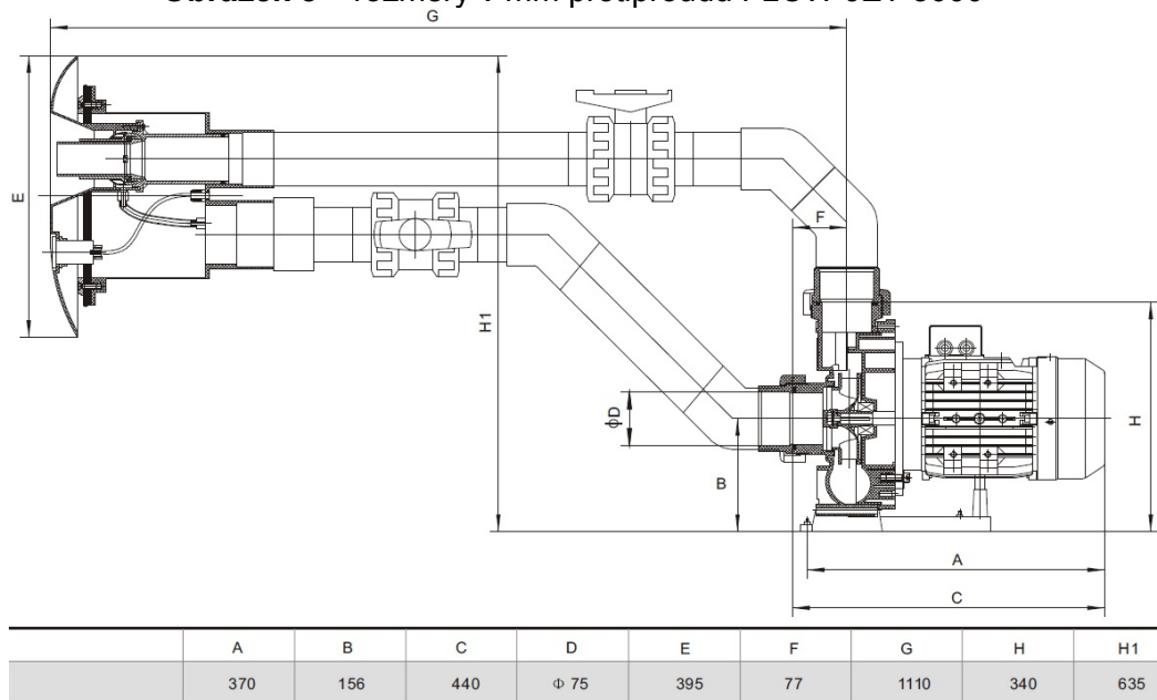
Obrázek 6 – rozměry v mm protiproudu FLOW JET 3000™
