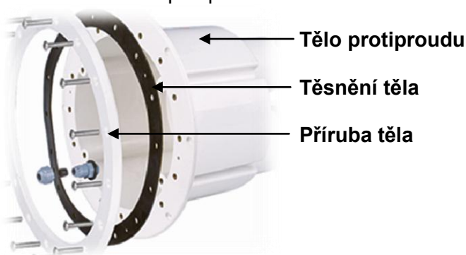
Obrázek 1 – tělo protiproudu
