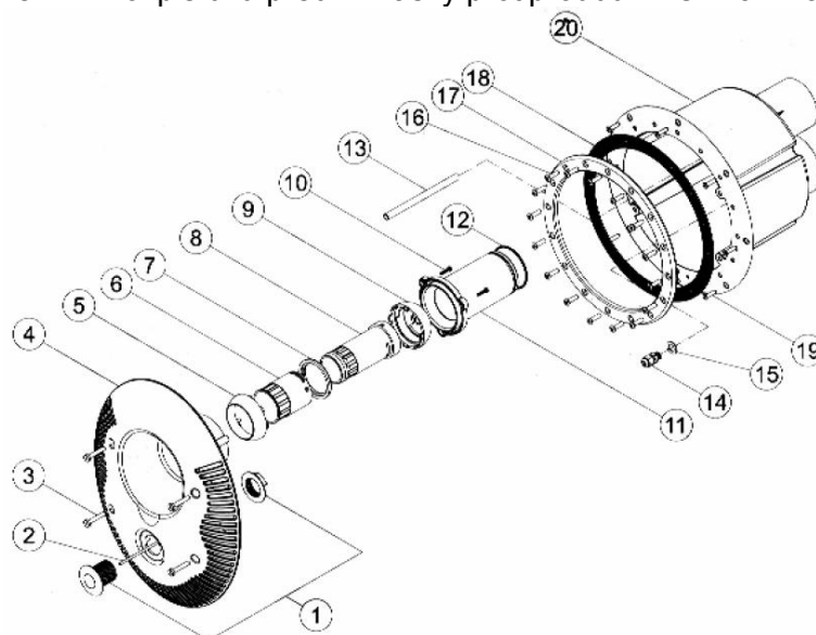
Obrázek 7 – rozpis dílů přední masky protiproudu FLOW JET 3000™
