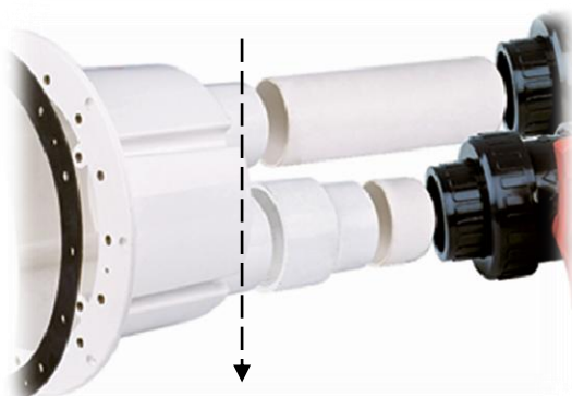
Obrázek 2 – tělo protiproudu musí být instalováno svisle: výtlač \varnothing 75 mm nad sáním \varnothing 90 mm
