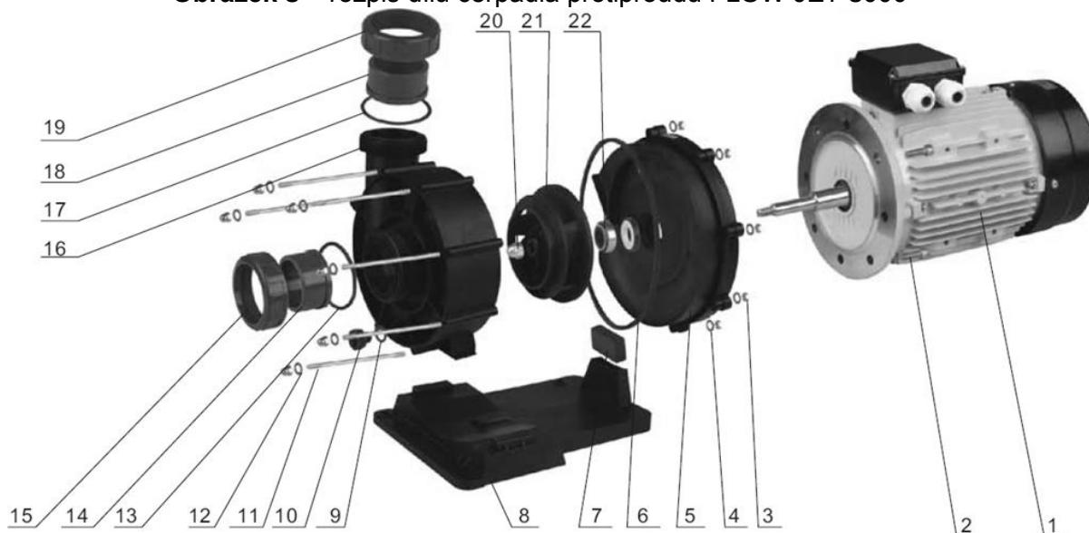
Obrázek 8 – rozpis dílů čerpadla protiproudu FLOW JET 3000™
