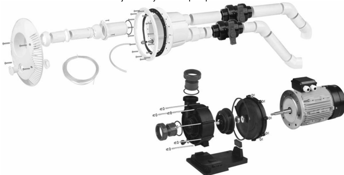
Obrázek 4 – rozkres jednotlivých částí protiproudu FLOW JET 3000™
